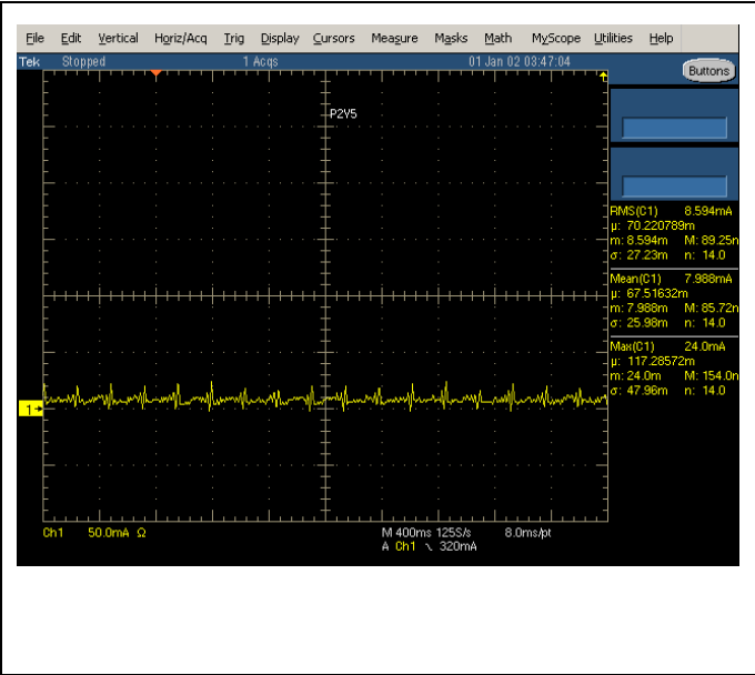
Fig. 8: P2V5
