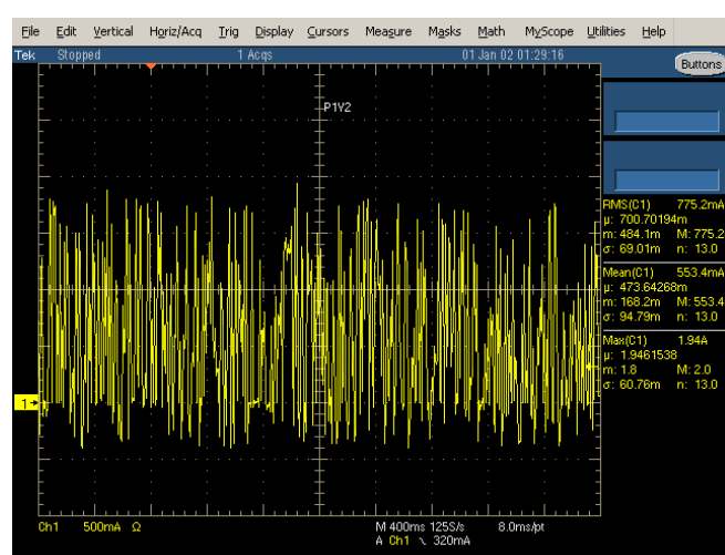
Fig. 2: VDD_EE
